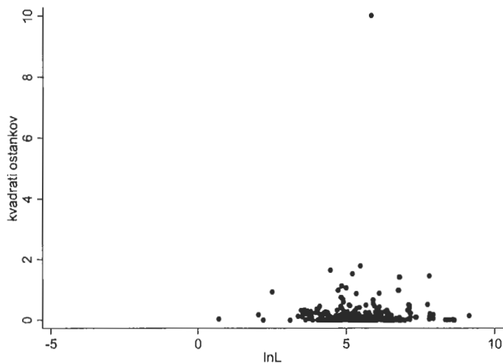
Slika 9: Kvadrati ostankov v odvisnosti od \ln L
