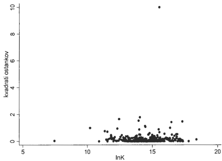
Slika 10: Kvadrati ostankov v odvisnosti od \ln K
